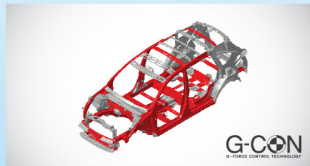
โครงสร้างตัวถังเบาะ G-CON และ ACE™ ปกป้องห้องโดยสารจากการชนรถที่ตก
